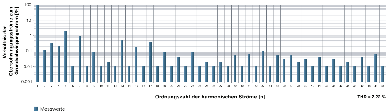
Oberschwingungsströme bei Nennleistung SolarMax 330TS-SV
