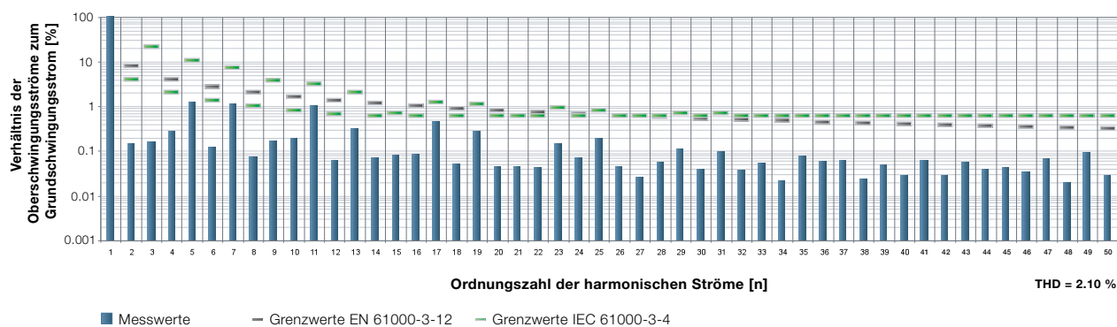
Oberschwingungsströme bei Nennleistung SolarMax 13MT2 / 13MT3
